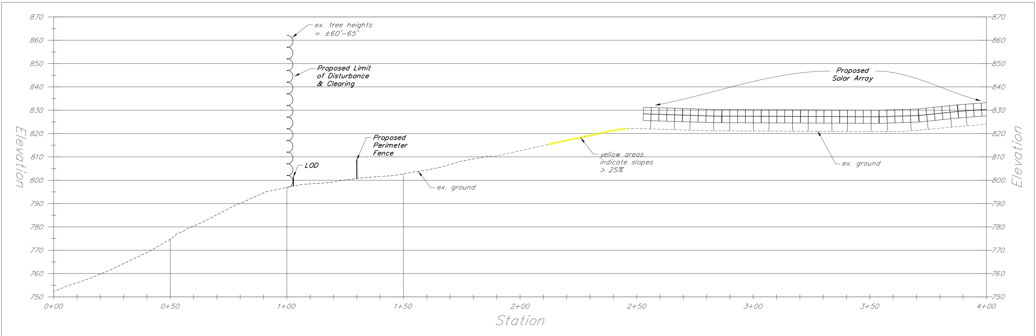
SECTION A-A (Sta. 0+00 - Sta. 4+00) HORIZONTAL & VERTICAL SCALE: 1"=20'
