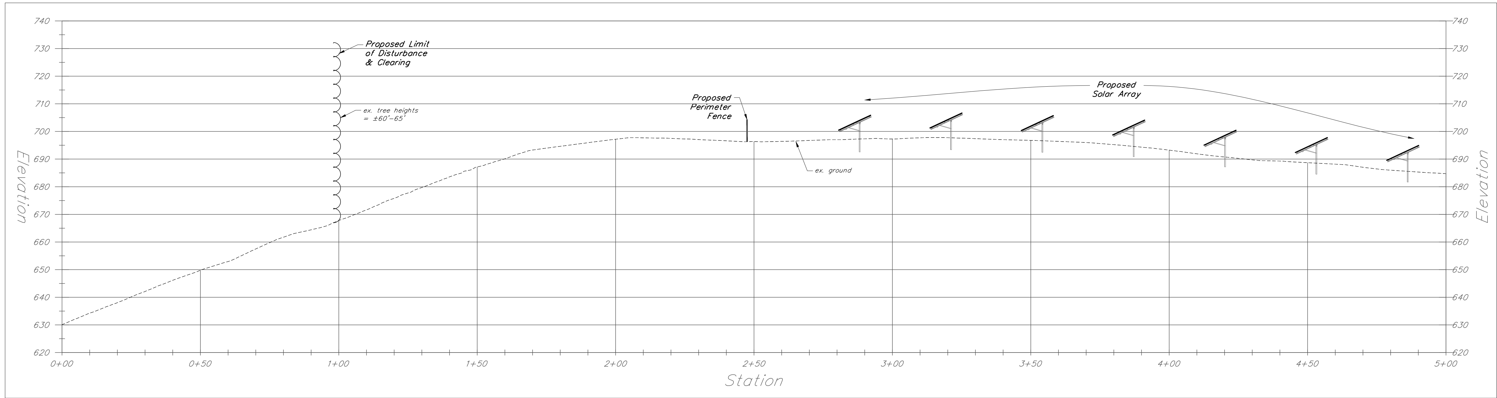
SECTION B-B (Sta. 0+00 - Sta. 5+00) HORIZONTAL & VERTICAL SCALE: 1"=20'
