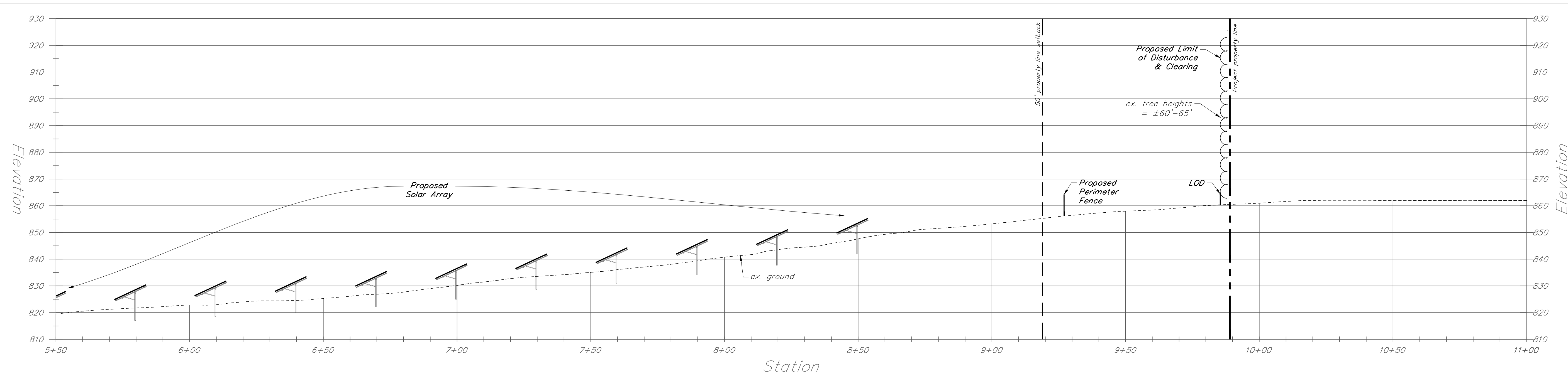
SECTION B-B (Sta. 5+50 - Sta.11+00) HORIZONTAL & VERTICAL SCALE: 1"=20'
