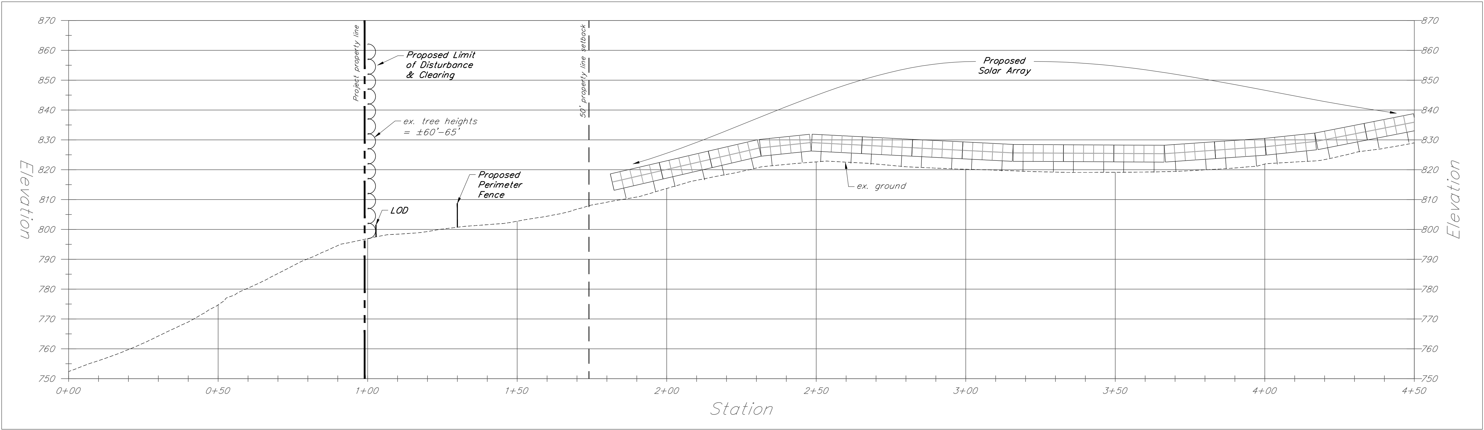
SECTION A-A (Sta. 0+00 - Sta. 4+50) HORIZONTAL & VERTICAL SCALE: 1"=20'
